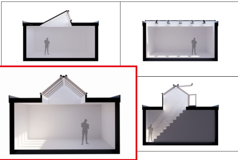
Lucernario a due falde
