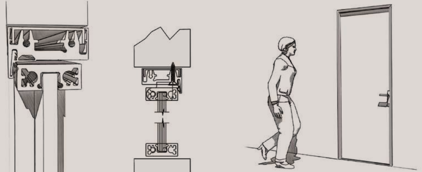
Telaio in alluminio minimale "MINIMALE" Anta singola "iINDUSTRIAL" battente con profilo in alluminio Mod.TRASPARENTE
