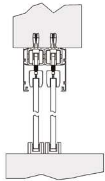
Sistema scorrevole con mantovana in alluminio SC5010_SC5010S Due ante parallele Fissaggio a soffitto o a parete
