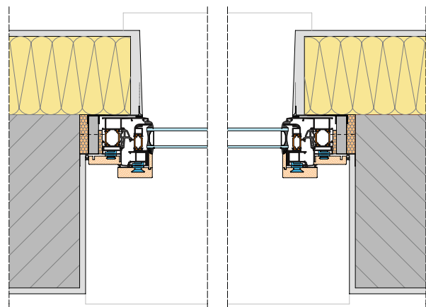
sezione orizzontale
