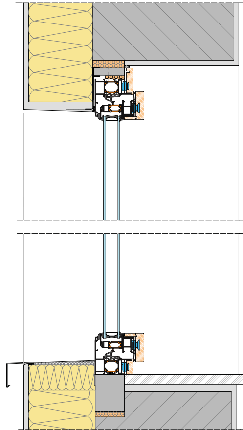
sezione verticale
