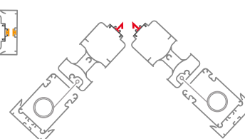
ANTA ANGOLARE
