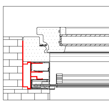
SEZIONE ORIZZONTALE
