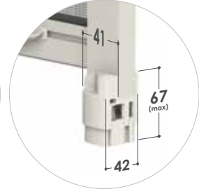
Piedini ad espansione di serie, apertura massima
