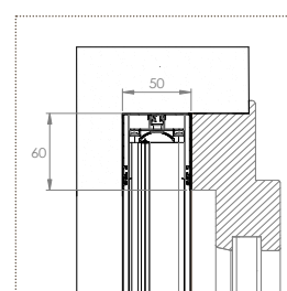
■ BORA INCAS STANDARD DOPPIA 20/20
