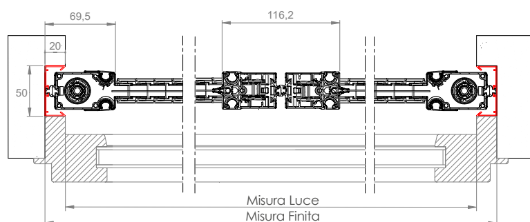
LINDAPLUS INCAS DOPPIA
