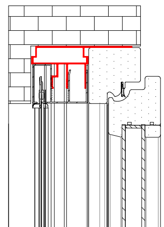
SEZIONE VERTICALE
