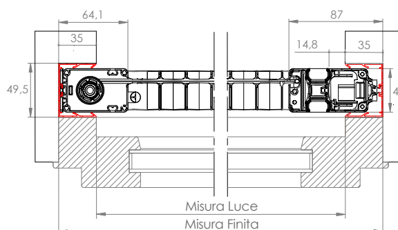
■ BORA INCAS MIDI 35/35
