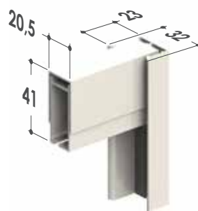
Guide telescopiche regolabili
