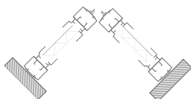
SEZIONE ANGOLARE
