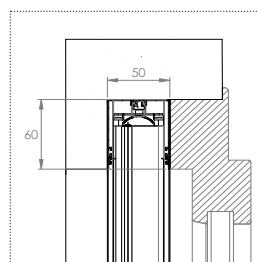
■ BORA INCAS STANDARD DOPPIA 35/35
