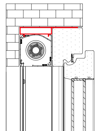
SEZIONE VERTICALE
