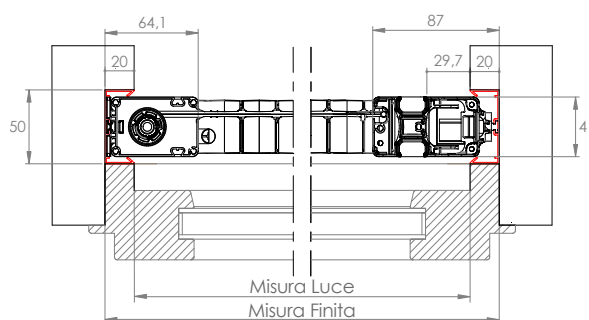
■ BORA INCAS MIDI 20/20
