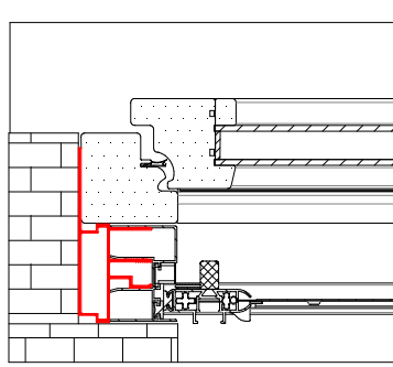
SEZIONE ORIZZONTALE
