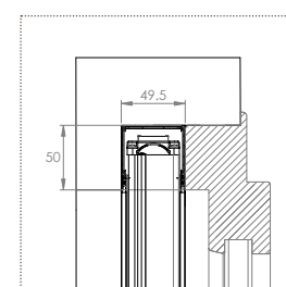
■ BORA INCAS MIDI DOPPIA 20/20
