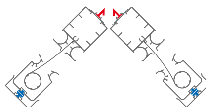
ANTA ANGOLARE
